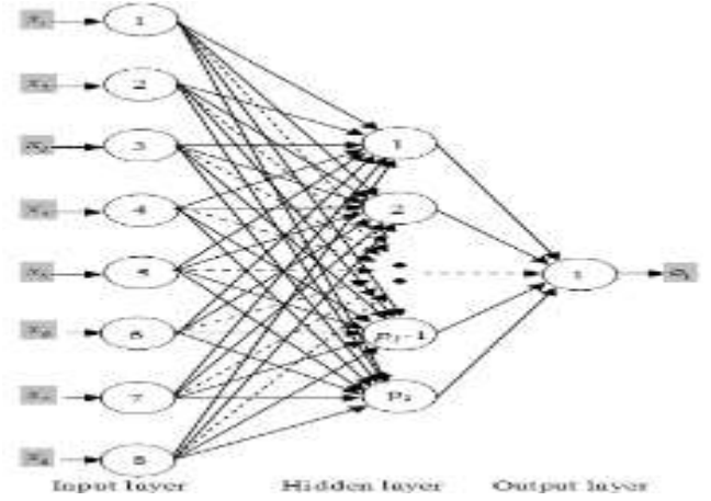
Fig. 1. ANN Model
